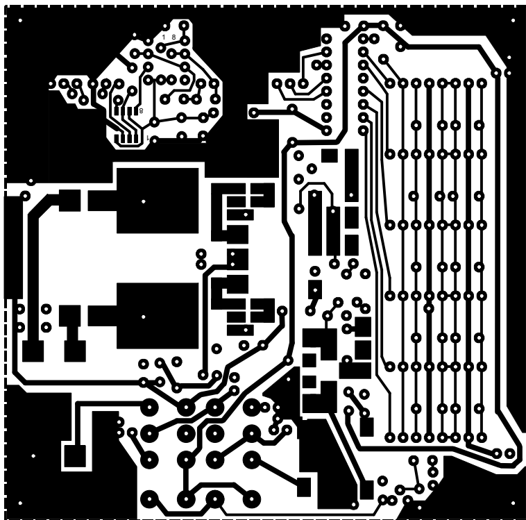
strona elementów - widok lustrzany
