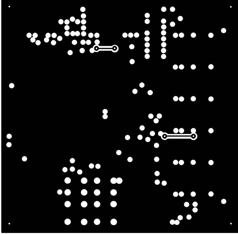
strona masy - widok prosty
