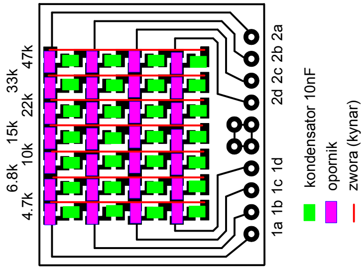
schemat montażowy filtra polifazowego
