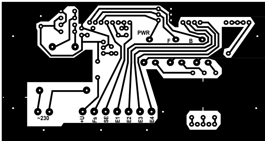
płytki przejściowa
